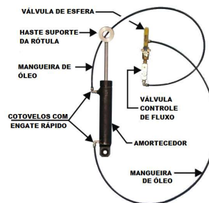
Amortecedores
